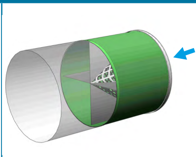
EQ - kužel z perforované tkaniny s hvězdicovitými příčnickami
