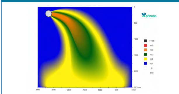
Obráz proudění, mikroperforace 90°, 165 Pa
