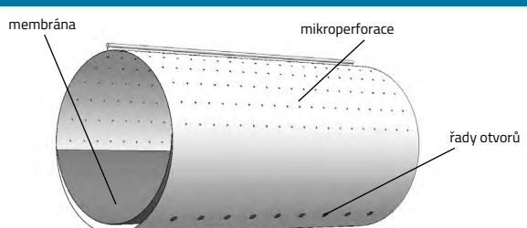
Schéma membránové výústky
