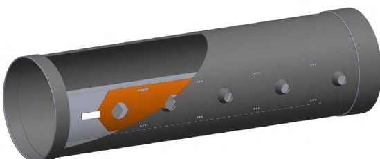
Možnost zaslepení některých trysek
