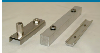
Zesílený hliníkový profil (I)
