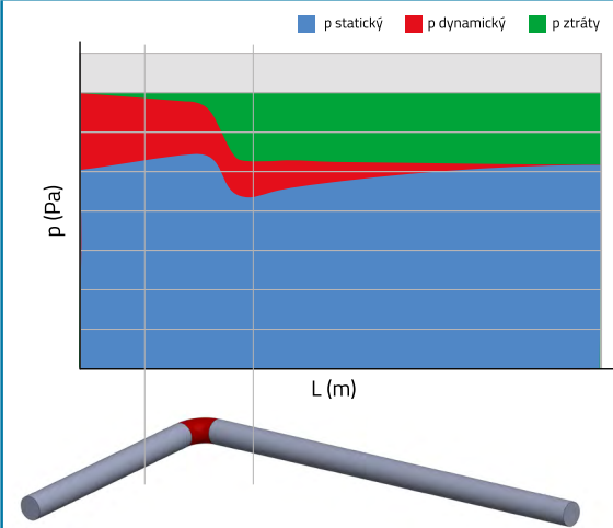
Graf rozložení tlaku v tkaninové výústce
