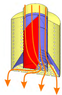
Lodret lufttilførsel
