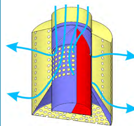
Vandret lufttilførsel
