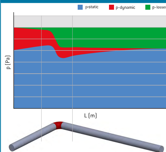
Graf for trykfordeling i tekstilbaseret system
