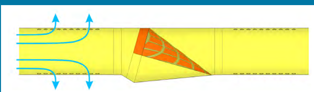
Lukket spjæld
