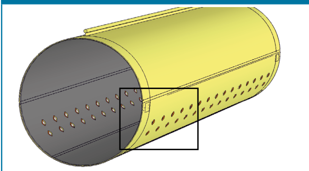
Diffusor med justerbar perforering
