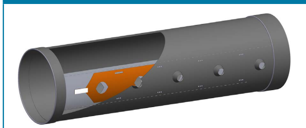
Mulighed for at afspærre visse dyser
